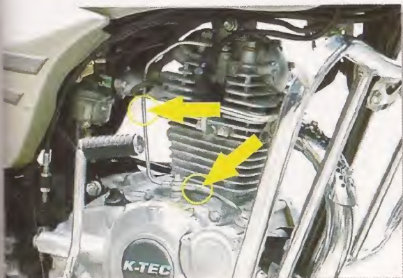
Mangueras de lubricación
